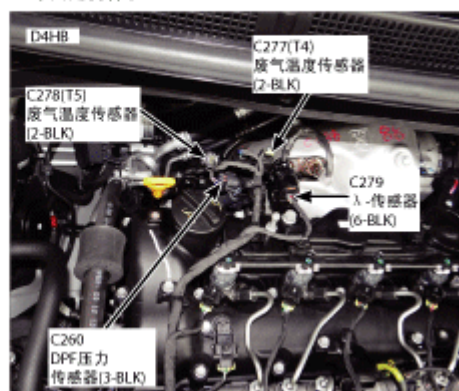
42.发动机右侧
