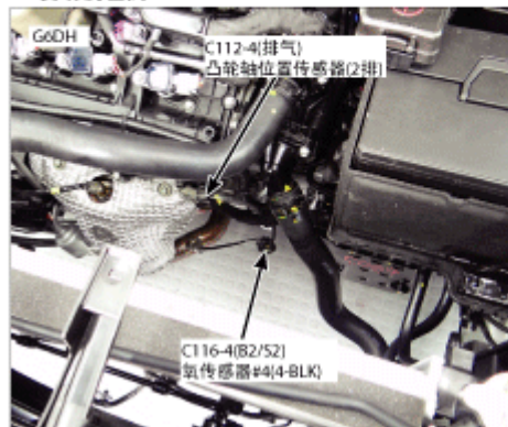
37.发动机左侧
