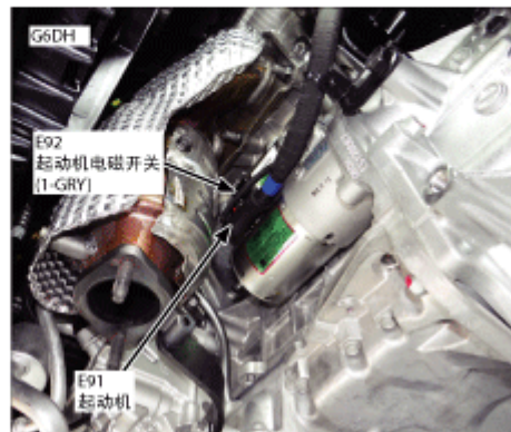
39.发动机左侧下部
