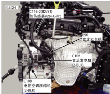
38.发动机左侧
