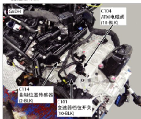
40.变速器顶部
